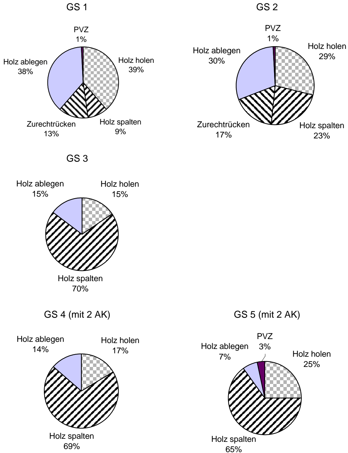
Abbildung 59: Zeitliche Verteilung der Arbeitsablaufabschnitte in den Große-Senkrechtspalter(GS)-Studien. Teilstudie GS 6 nicht dargestellt (keine einzelnen Ablaufabschnitte gemessen). AK Arbeitskräfte
