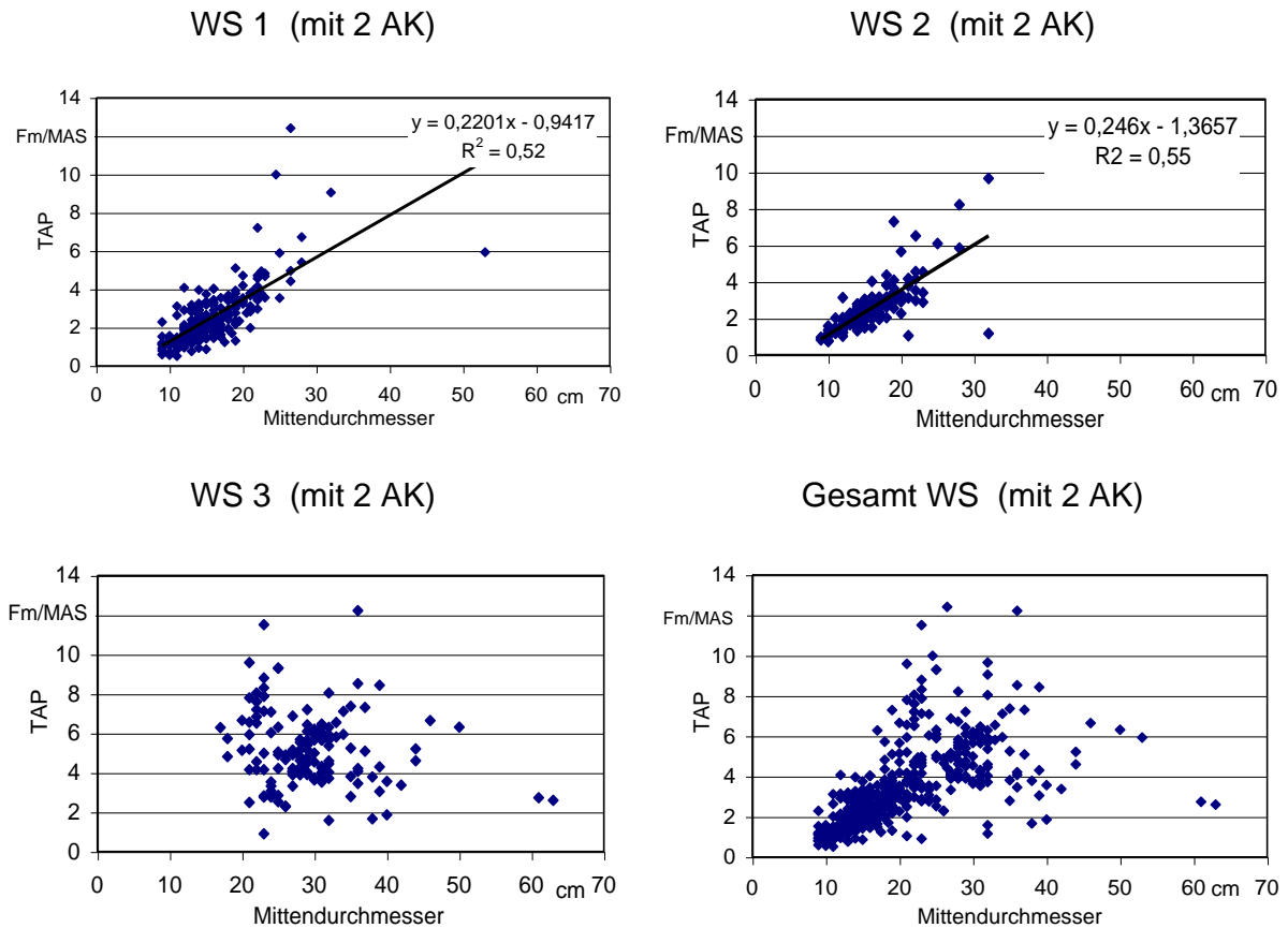
Abbildung 66: Technische Arbeitsproduktivität (TAP) je Maschinenstunde beim Einsatz des Waagrechtspalters (WS) in Abhängigkeit vom Mittendurchmesser der Rundlinge AK Arbeitskräfte
