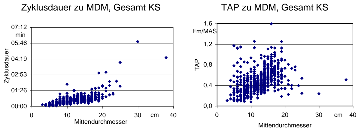
Abbildung 56: Zyklusdauer und technische Arbeitsproduktivität (TAP) in Abhängigkeit vom Mittendurchmesser (MDM) der Rundlinge (Werte aus allen Kleine-Senkrechtspalter(KS)-Studien)
