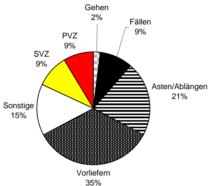
Abbildung 40: Zeitanteile Holzernte Teilstudie 4 (Fichte). PVZ: persönliche Verteilzeit, SVZ: sachliche Verteilzeit
