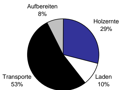
Abbildung 117: Endenergieverbrauchsanteile verschiedener Phasen der Scheitholzbereitstellung, dargestellt für die vier ausgewählten Modellverfahrensketten. Holzernte: Holzerte und Rücken. Transporte: Hin- und Zurück Wald-Bearbeitungsplatz-Kunde. Laden: Be- und Entladen und Aufschichten des Holzes. Aufbereiten: Ablängen, Spalten, Beschicken
