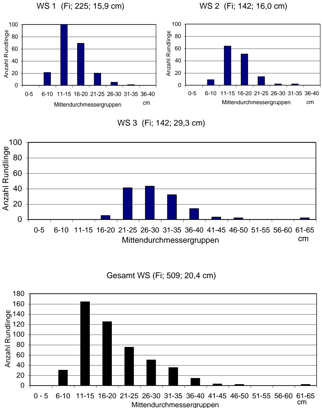
Abbildung 63: Die Verteilung der Mittendurchmesser des Holzes in den Waagrechtspalter(WS)-Studien. Grafiktitel mit Baumart, Anzahl Rundlingen und mittlerem Mittendurchmesser
