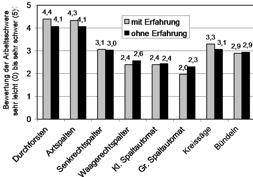
Abbildung 79: Ergebnisse der Befragung zur Einschätzung der Arbeitsschwere; Einteilung von sehr leicht (0) bis sehr schwer (5). Beim Senkrechtpaltern erfolgte keine Differenzierung in große oder kleine Geräte
