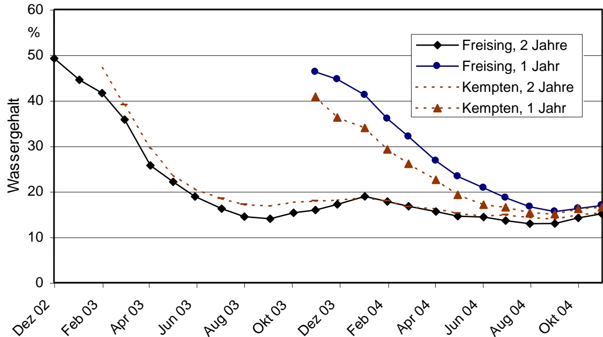
Abbildung 97: Vergleich des Trocknungsverlaufes von Buchenscheitholz an den Standorten Freising und Kempten. Lagerart: außen, abgedeckt, gespalten
