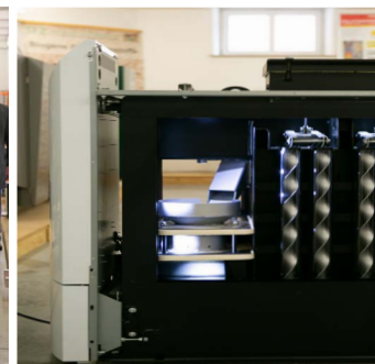
Schnittmodell eines Pelletkessels mit Wirbulatoren und Brennertopf
